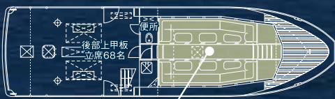
船体概要
